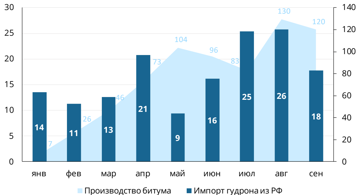
Динамика поставки гудрона и производства битумов в РК, январь-сентябрь 2023г, тыс. т. 1
