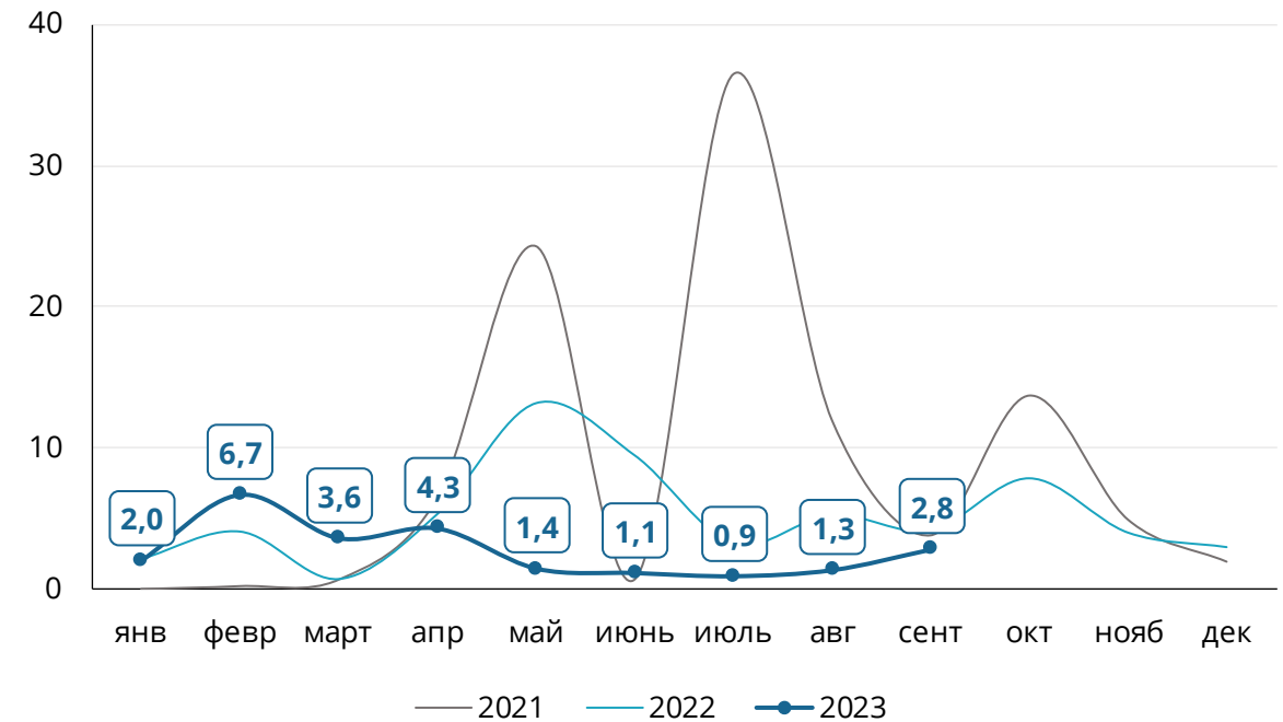
Динамика экспорта битумов из РК, январь-сентябрь 2021-2023гг, тыс. т.
